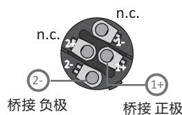
功率输出 1 桥接模式
