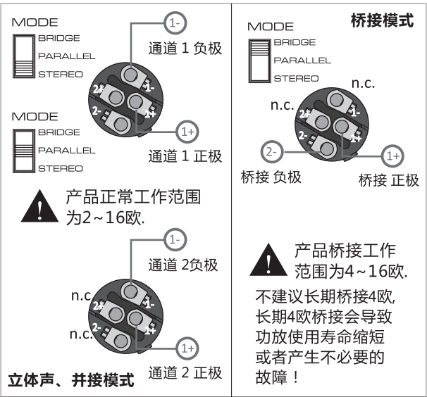
SPEAKON 功率输出 - 扬声器输出 NL4 Speakon 接线方式
