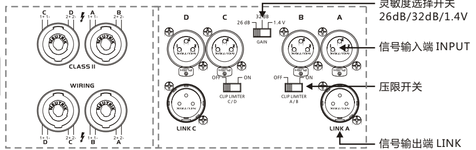
功率输出端
