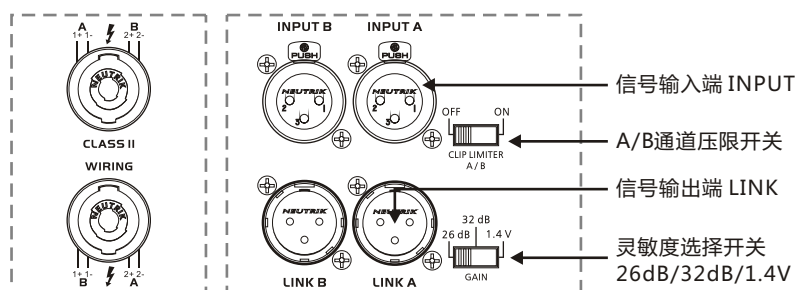
信号连接端
