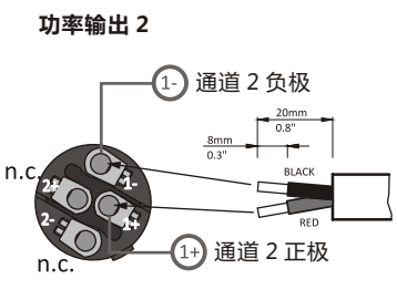
SPEAKON 功率输出 - 扬声器输出 NL4 Speakon 接线方式
