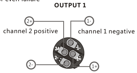
OUTPUT 1
