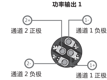
功率输出 1
