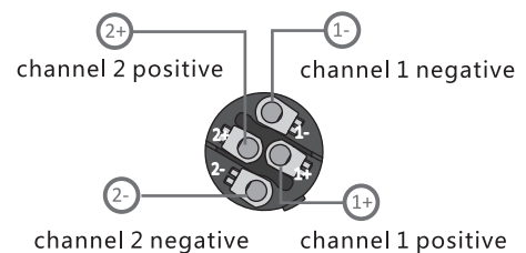
OUTPUT 1
