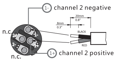
OUTPUT 2
