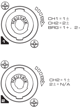
SPEAKON 功率输出 - 扬声器输出 NL4 Speakon 接线方式
