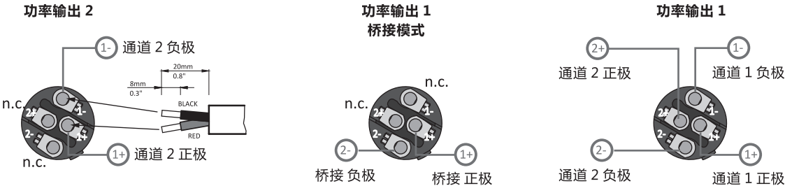
SPEAKON 功率输出 - 扬声器输出 NL4 Speakon 接线方式
