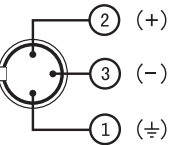
平衡XLR接线方式
