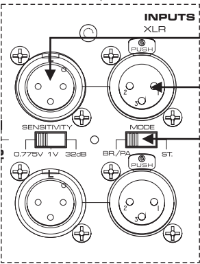
平衡XLR接线方式
