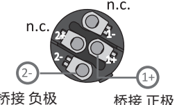
功率输出 1 桥接模式
