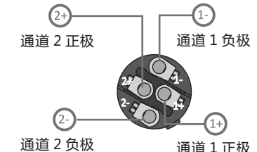
功率输出 1
