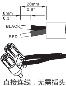
电源线
