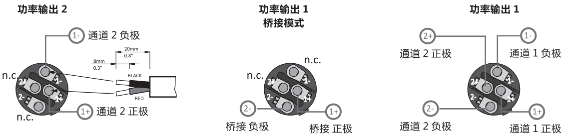
SPEAKON 功率输出 - 扬声器输出 NL4 Speakon 接线方式
