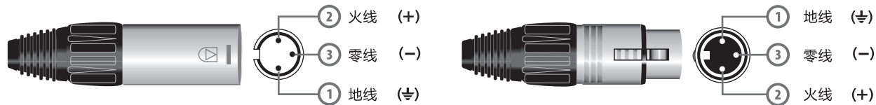
输入 INPUT 平衡连接 公座 XLR
