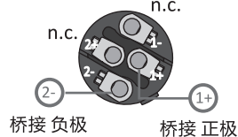
功率输出 1 桥接模式
