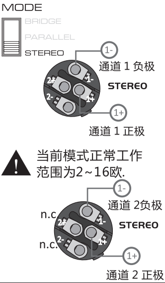
SPEAKON 功率输出 - 扬声器输出 NL4 Speakon 接线方式
