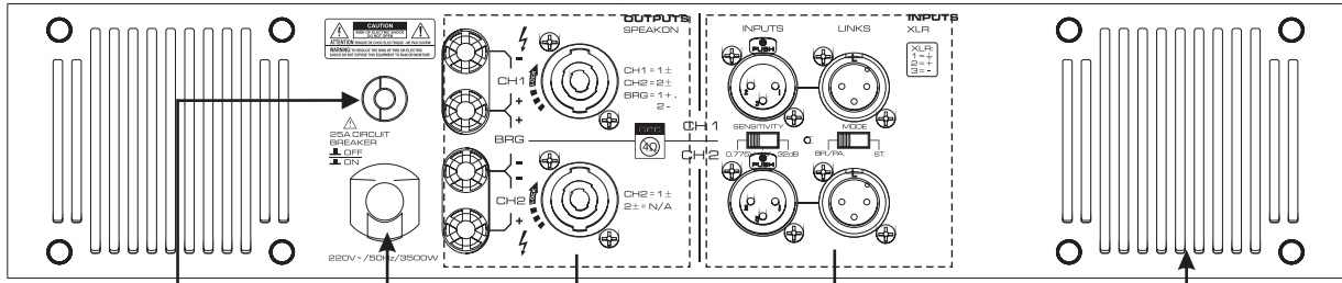
断路器 (VO08~VO36带保险管座的电源线插座) 电源线 功率输出端 信号连接端 排风扇
