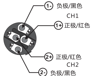
音箱螺旋插头 Speakon (NL4)
