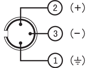
平衡XLR接线方式
