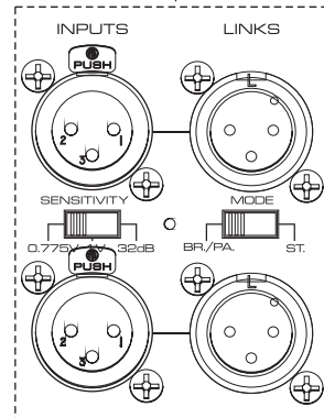
平衡XLR接线方式
