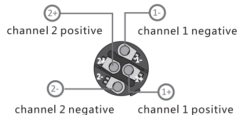
OUTPUT 1
